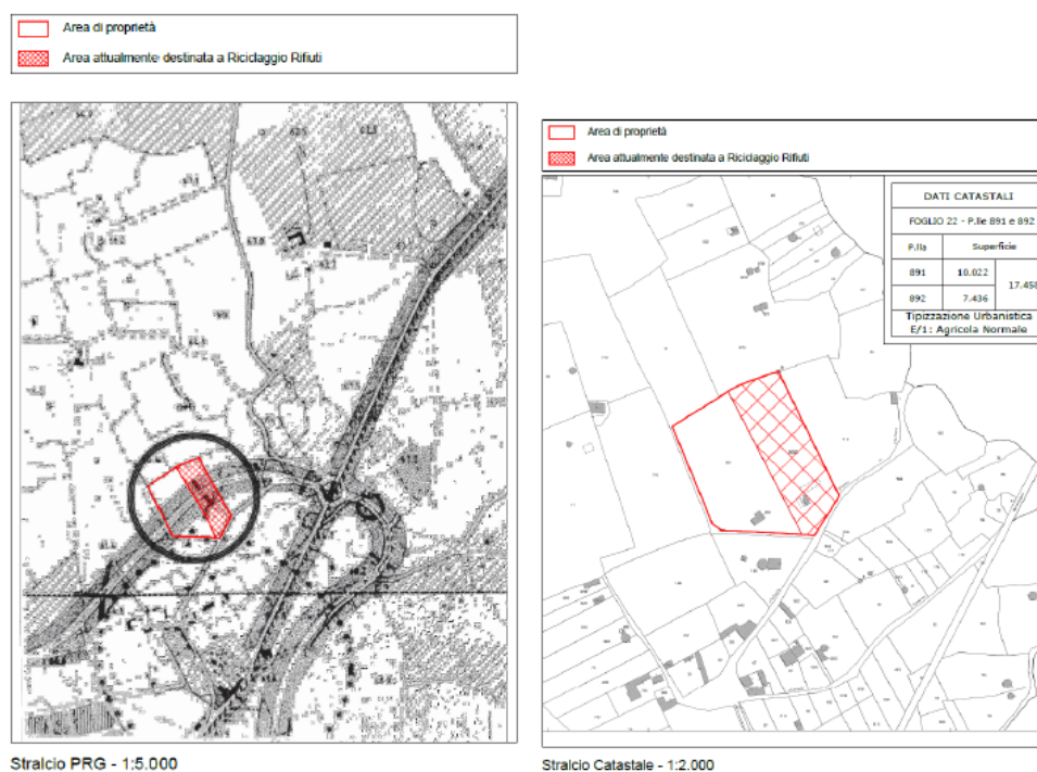
Fig. 2. Elaborato - VIA_01_Studio di impatto ambientale (tralcio PRG castale).
